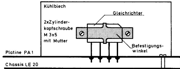
Abb. 4a: Montage des Gleichrichters
