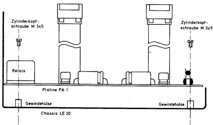
Abb. 7: Montage der PA 1 im Chassis LE 20
