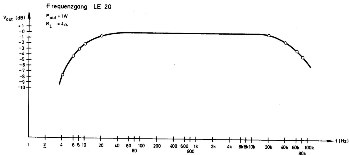
Kurve 1: Frequenzgang der Endstufen
