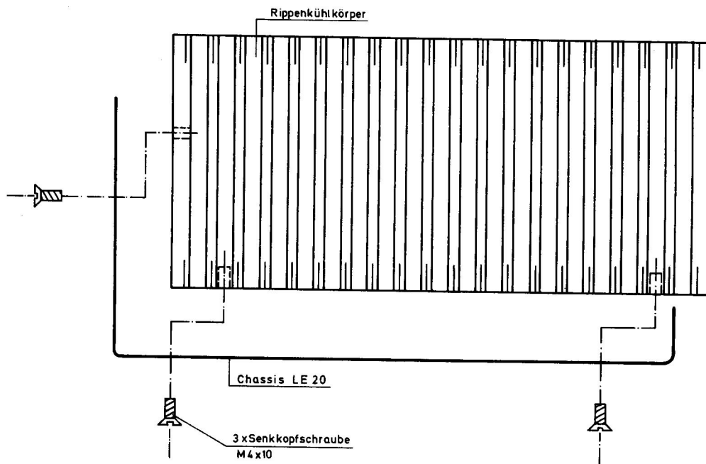
Abb. 9: Montage des Kühlkörpers am Chassis LE 20
