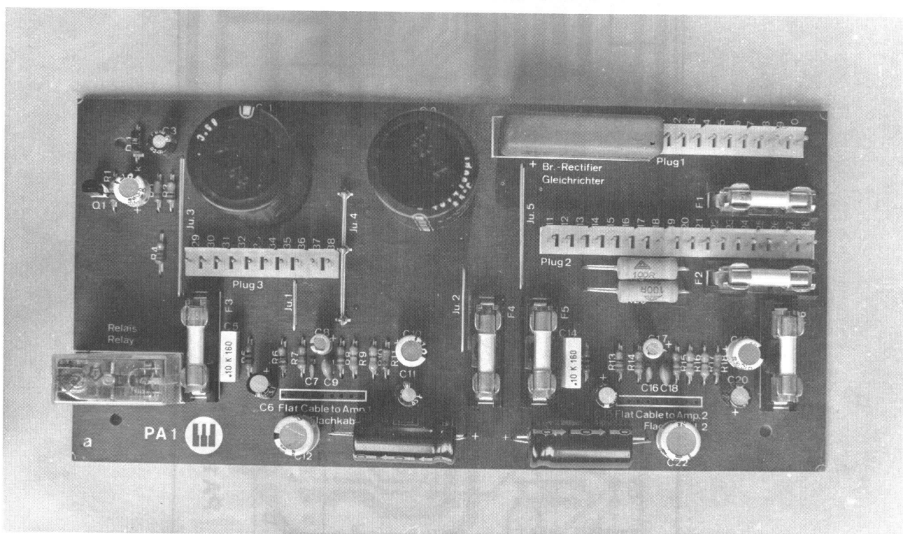
Abb. 4: Fertig bestückte Platine PA 1
