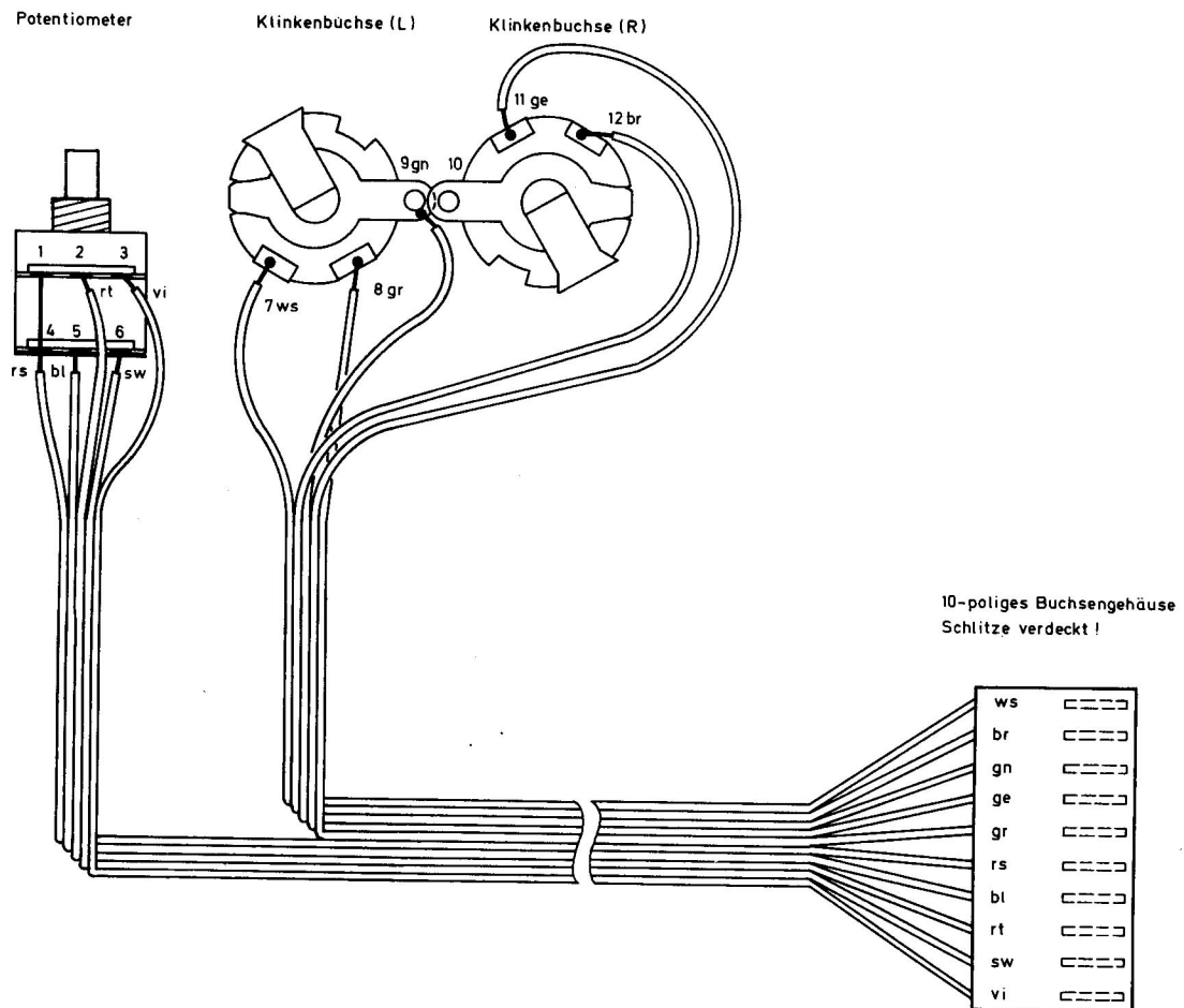
Abb. 6: Anschluß des 10-adrigen Flachkabels
