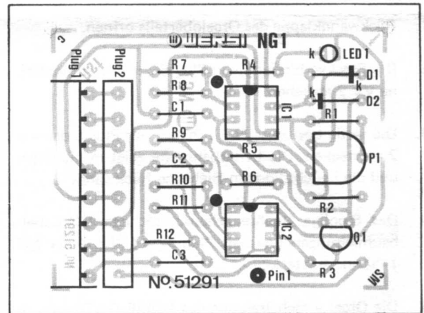
Abb. 2: Positionsdruck NG 1 mit gerastert unterlegten Leiterbahnen
