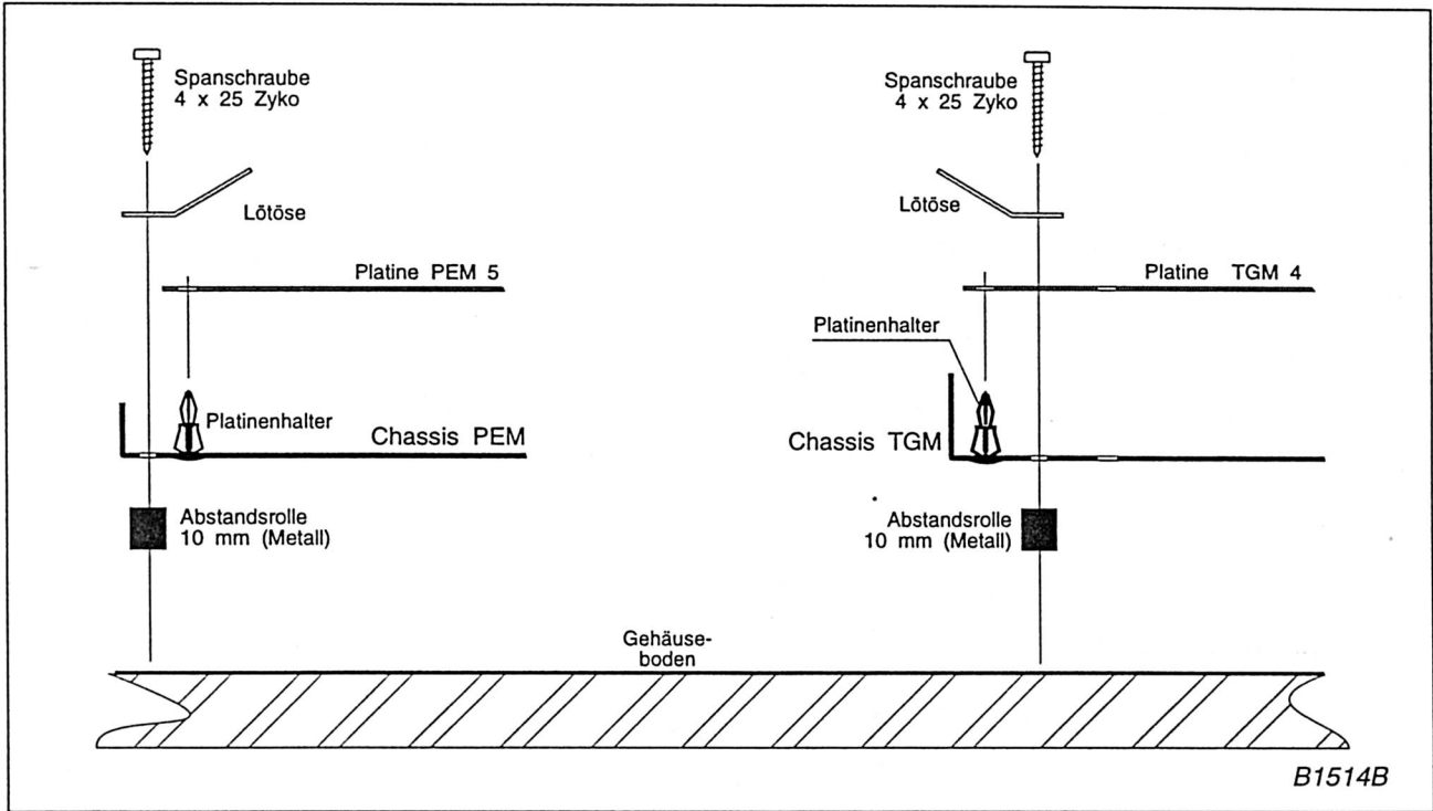
Abb. 9a: Vorbereitung und Befestigung der Metallchassis PEM und TGM
