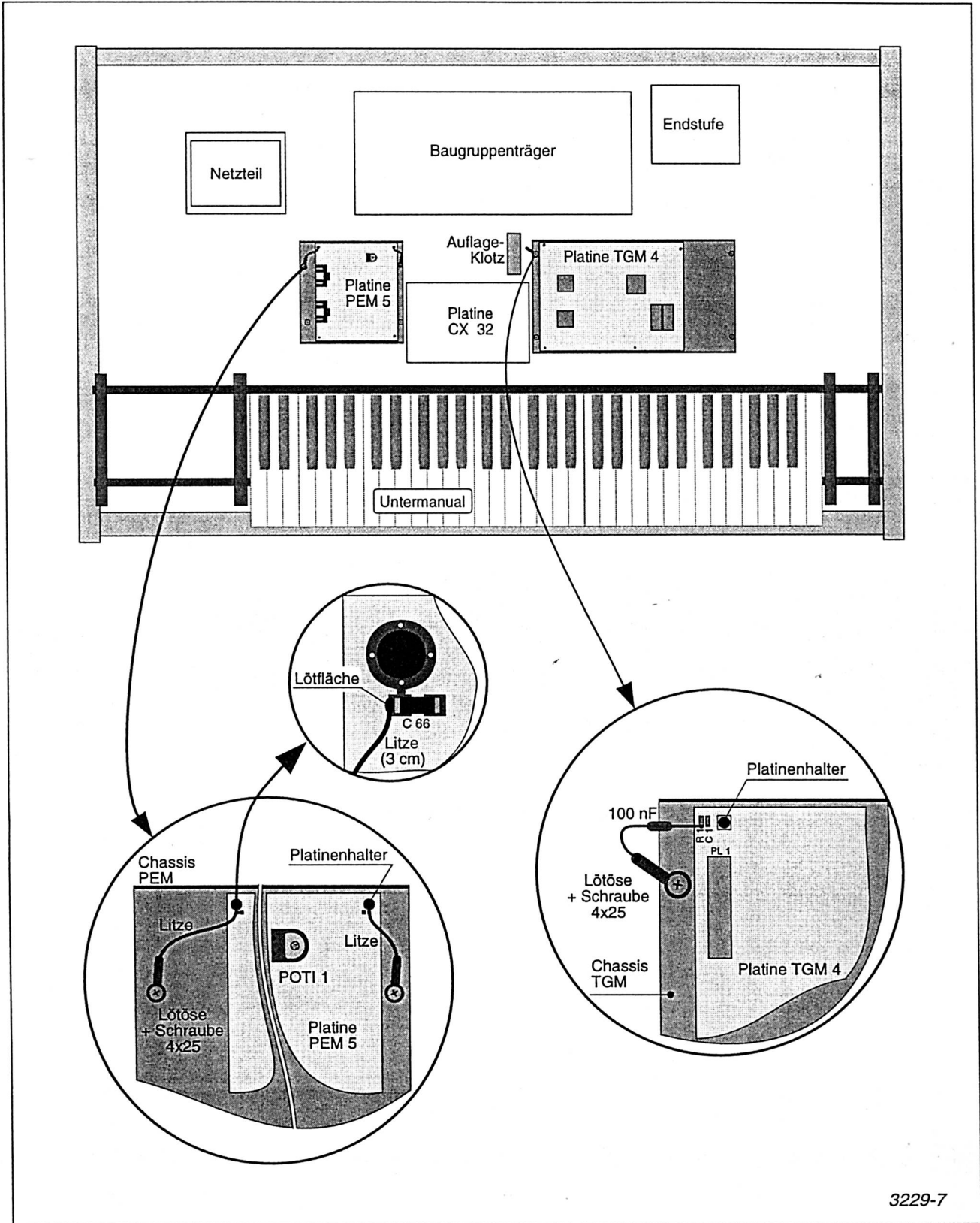
Abb. 11: Lage der Baugruppen in einer SPECTRA; bei anderen Modellen evtl. geringfügig abweichend
