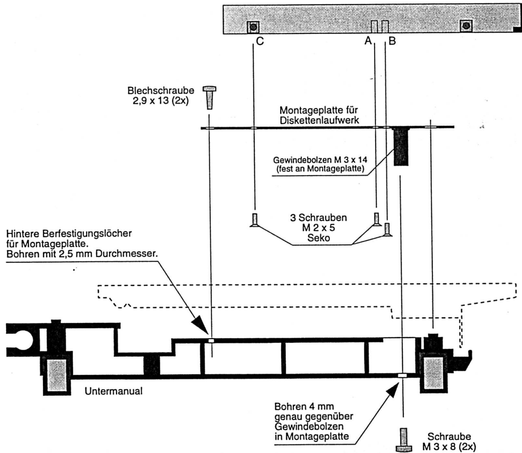
Diskettenlaufwerk, Seitenansicht
