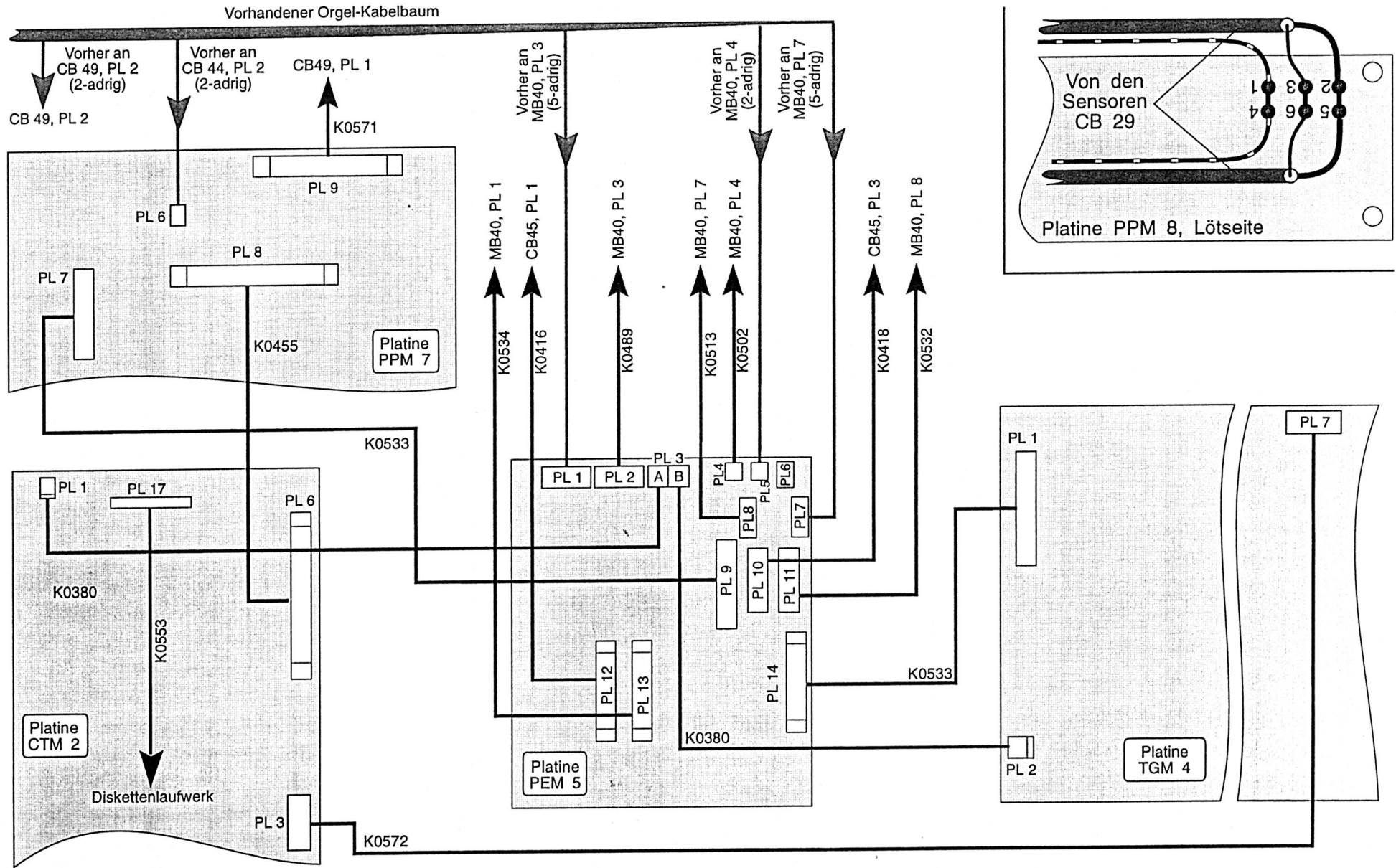
Abb 12: Verdrahtung der GOLDEN GATE, schematisch
