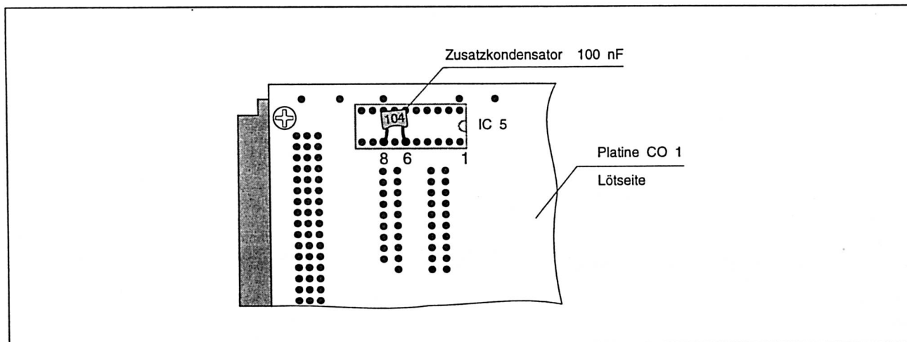
Abb. 17: Zusatzkondensator auf der Lötseite der Platine CO 1
