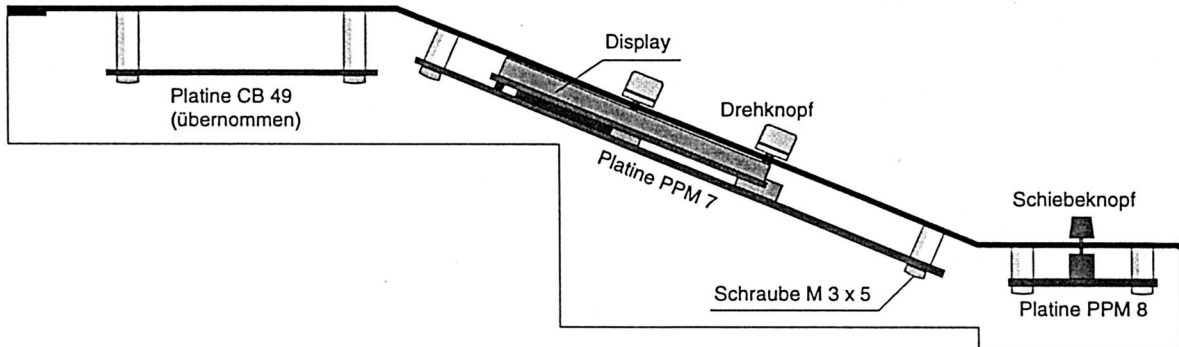
Bedienfeld links (Blech), Seitenansicht
