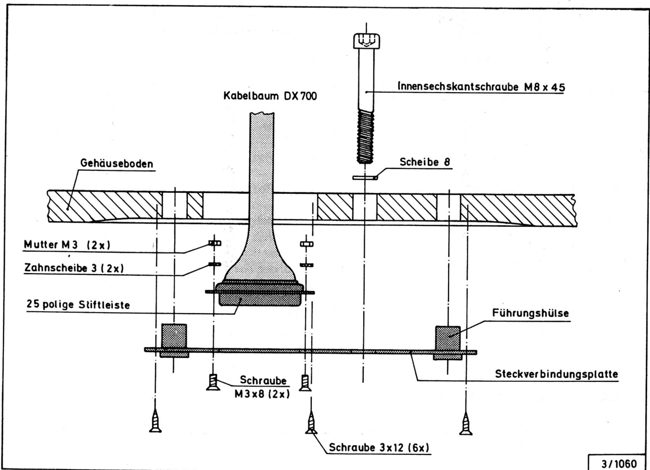
Abb. 10: Steckverbindung und Kabelbaum, rechts
