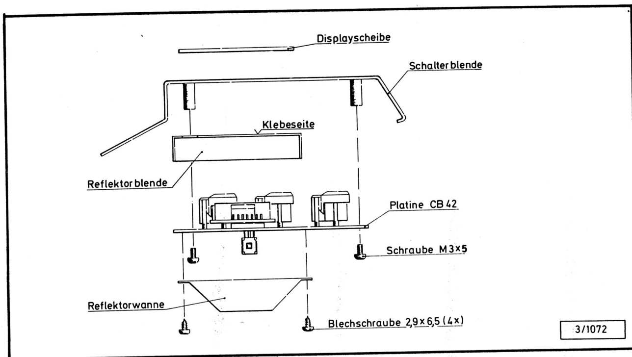
Abb. 8: Montage der Display-Abdeckscheibe
