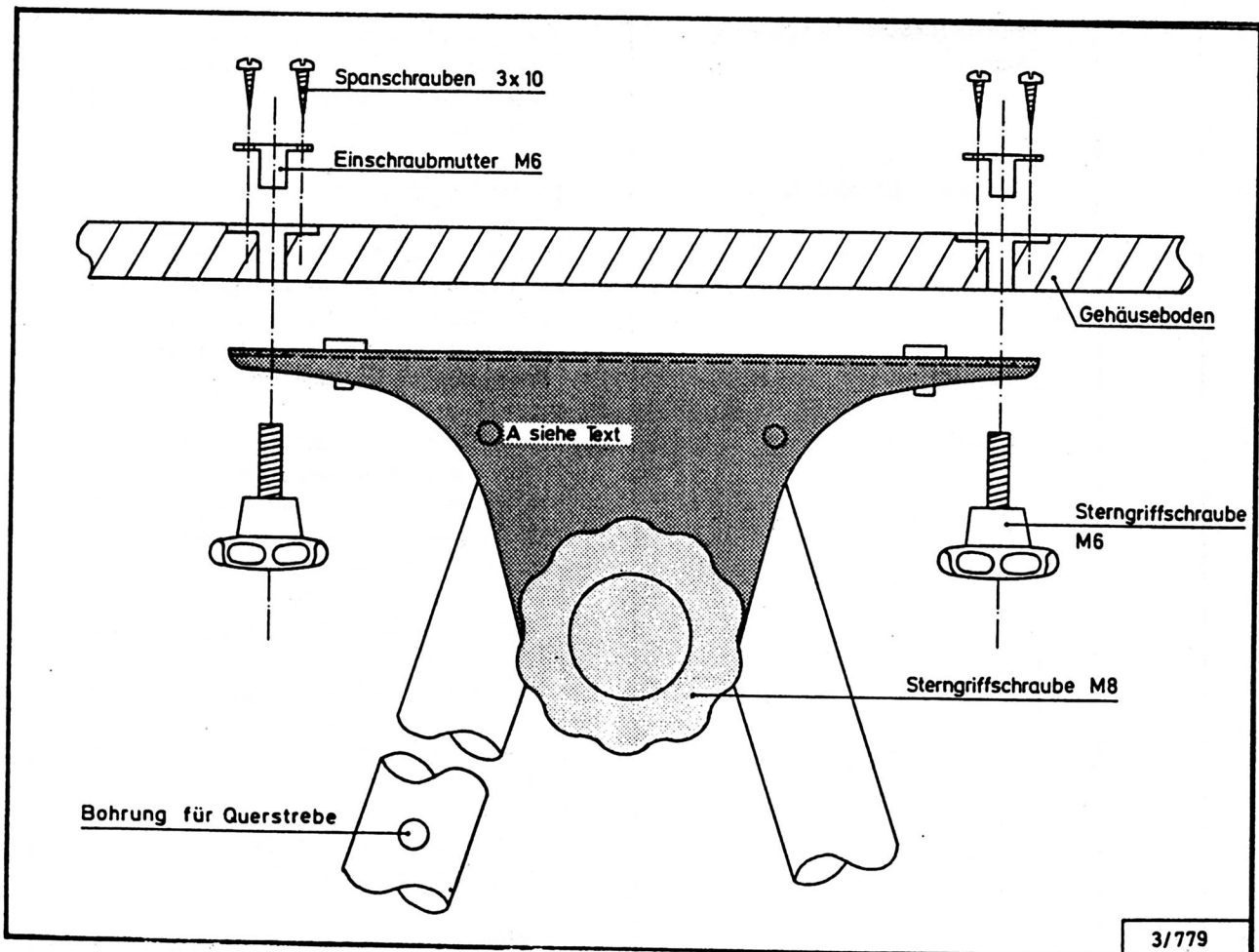
Abb. 16: Aufbau des verchromten Fußgestells
