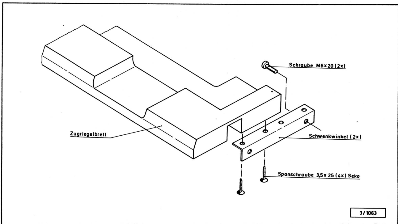
Abb. 6: Einbau des Zugriegelbrettes
