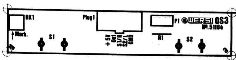
Abb. 14: Positionsdruck Platine OS 3
