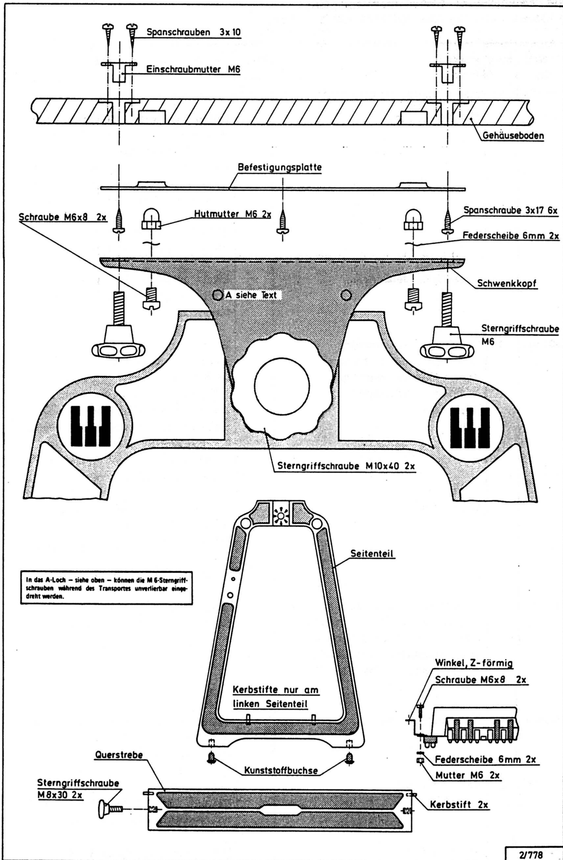
Abb. 17: Aufbau des Alu-Fußgestells
