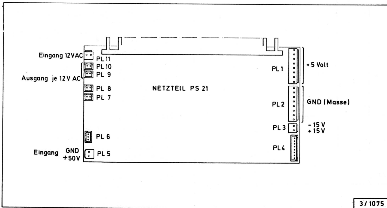
Abb. 18: Sollspannungen am Netzteil PS 21
