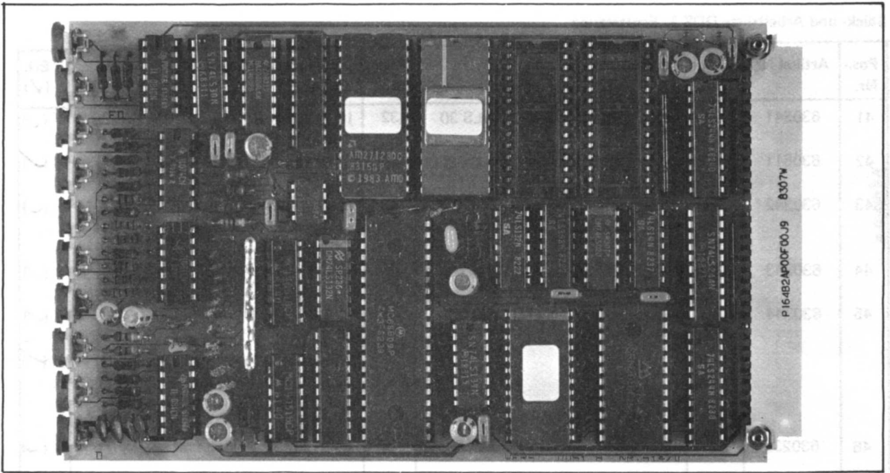
Abb. 10: Fertig bestückte Steckkarte DDS 1
