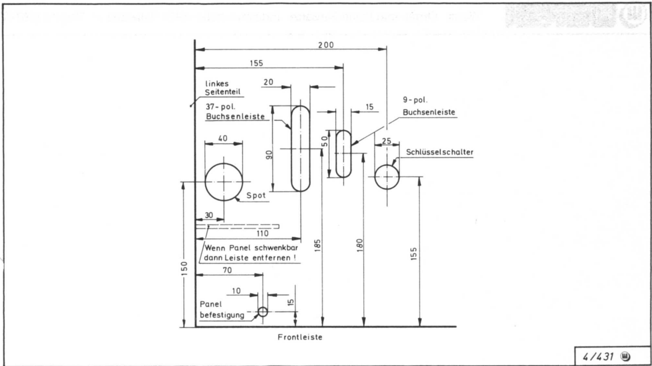
Abb. 49c: Maßskizze zum Paneleinbau in W 3 T
