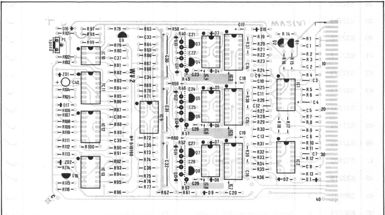
Abb. 43: Positionsdruck und Leiterbahnen WV 2
