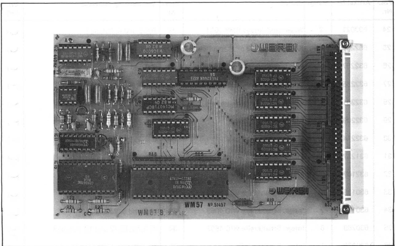
Abb. 38: Fertig bestückte Steckkarte WM 57
