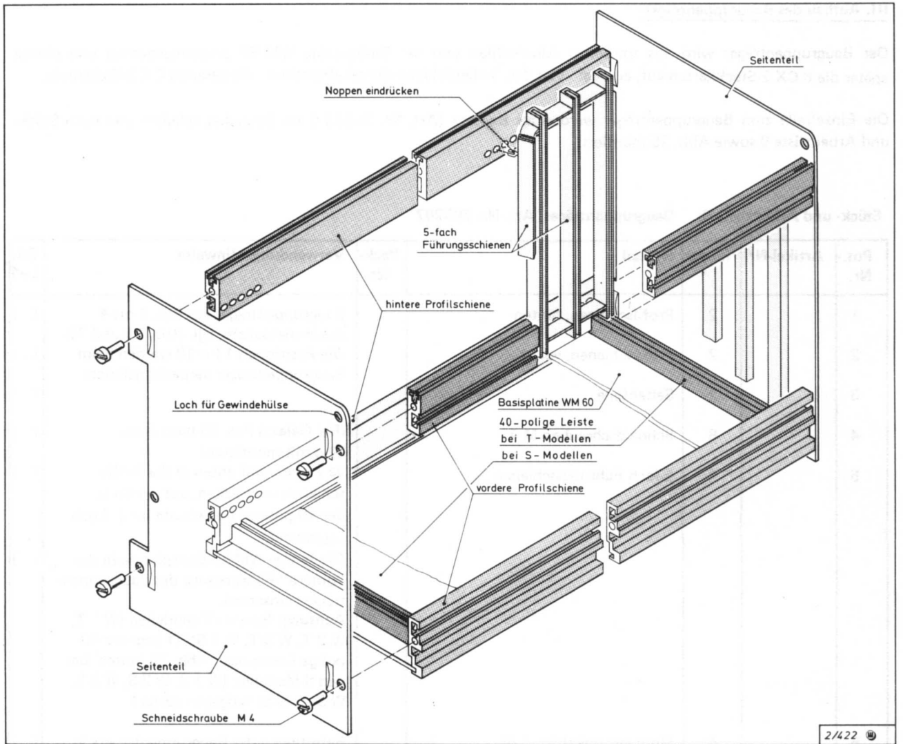
Abb. 25: Aufbau des Baugruppenträgers
