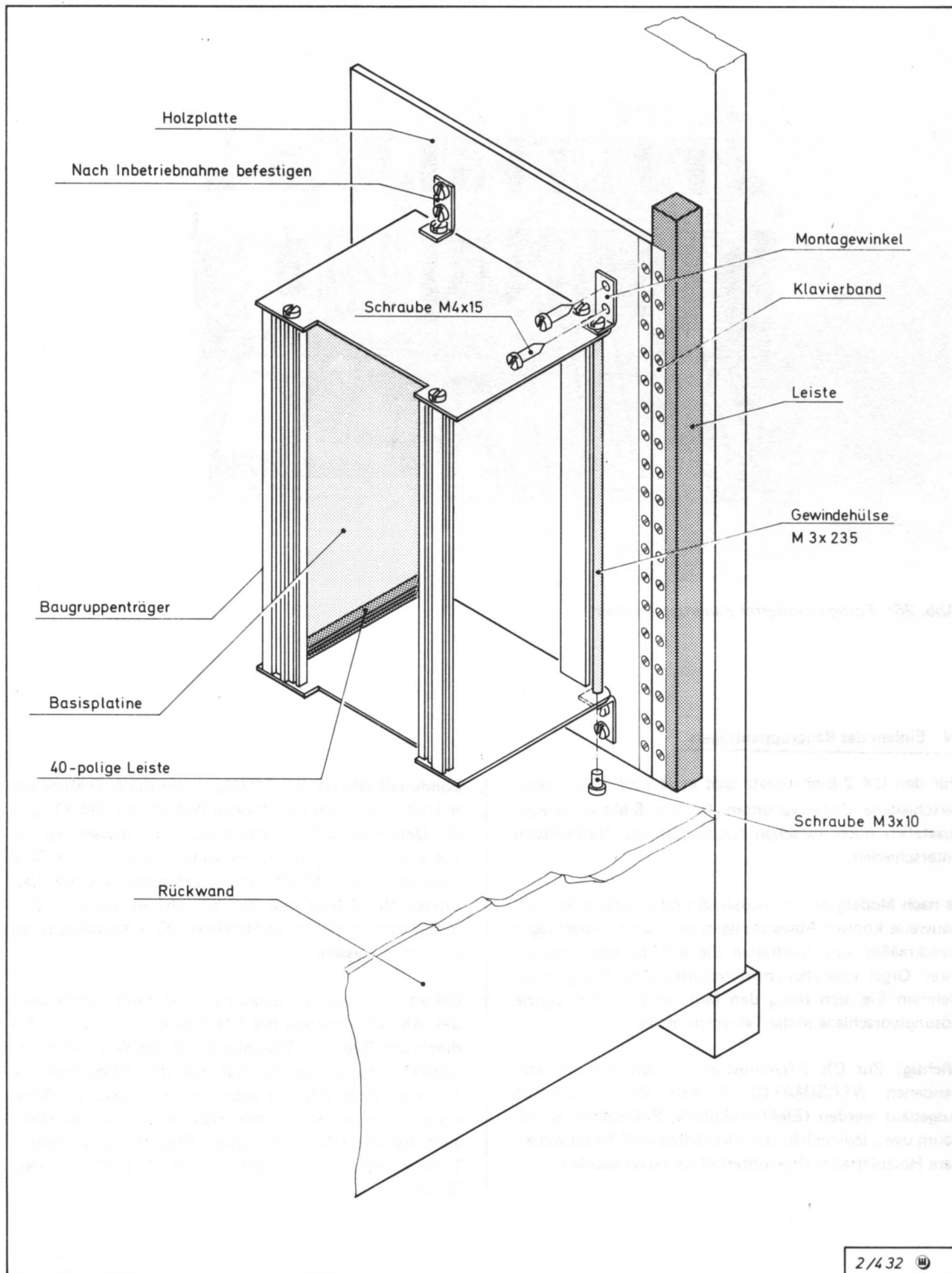
Abb. 27a: CX 2-Nachrüstung in W 1 S, W 2 S, W 3 S und W 3 A
