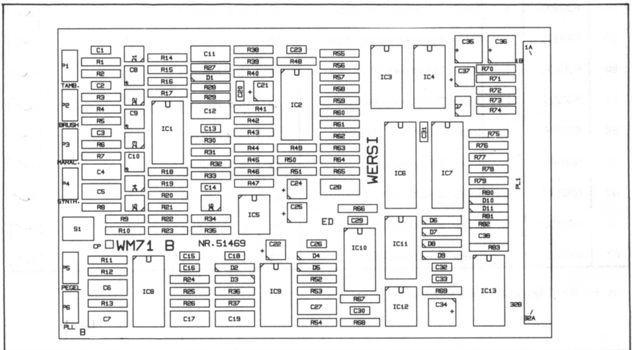
Abb.9: Positionsdruck WM 71
