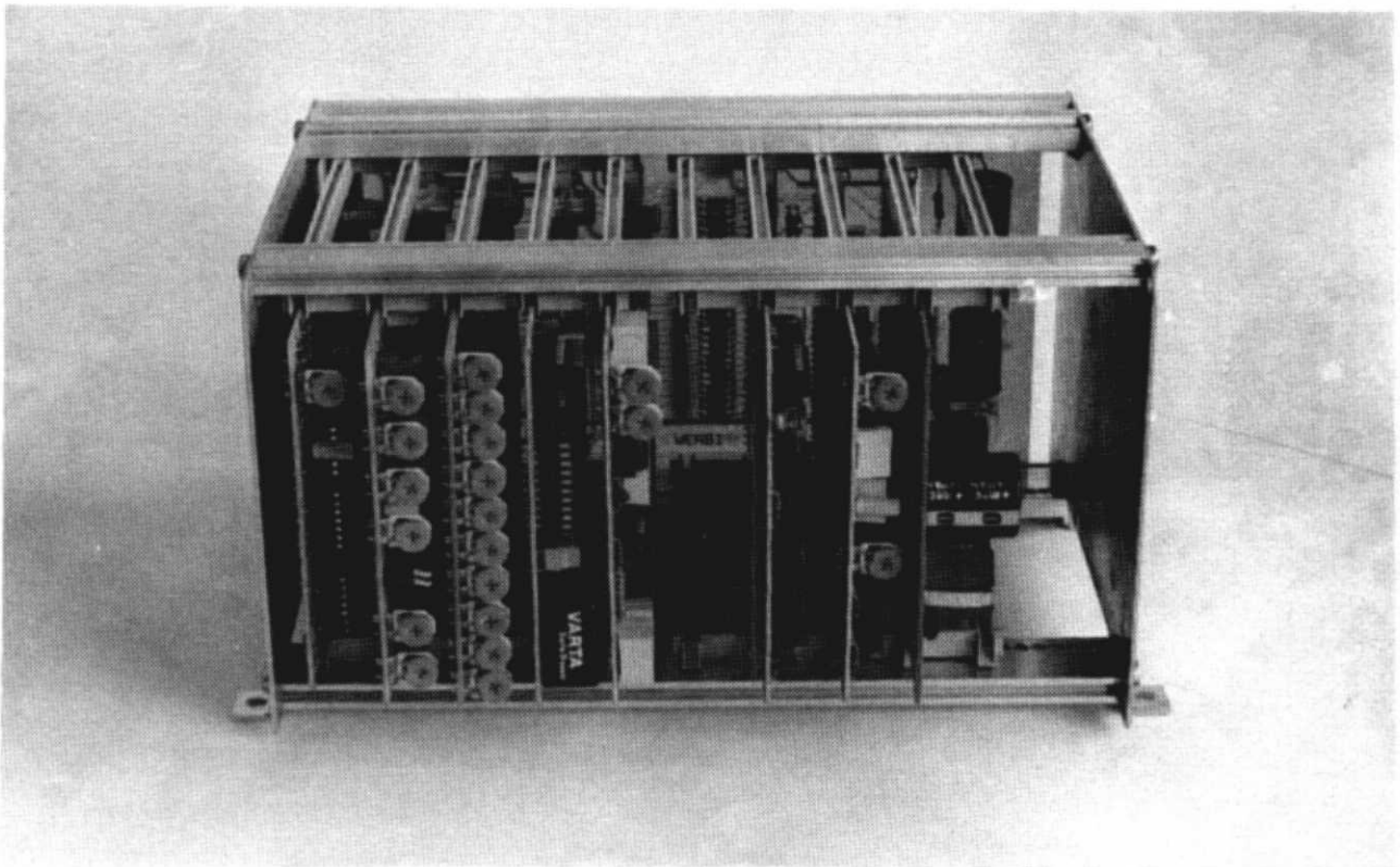
Abb. 1: Hardware CX 2 (Foto Baugruppenträger mit Steckkarten)
