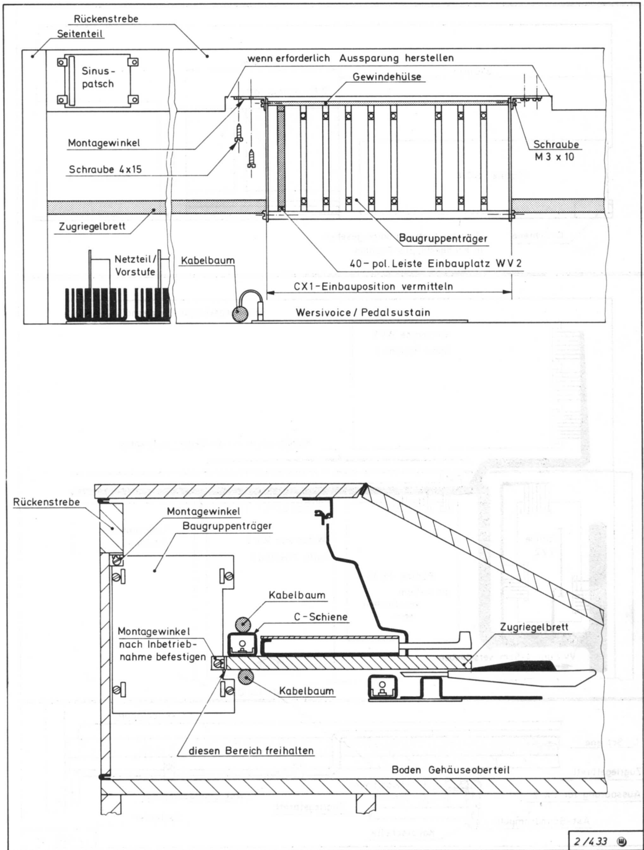
Abb. 27d: CX 1 in W2 T/TV und W3 T
