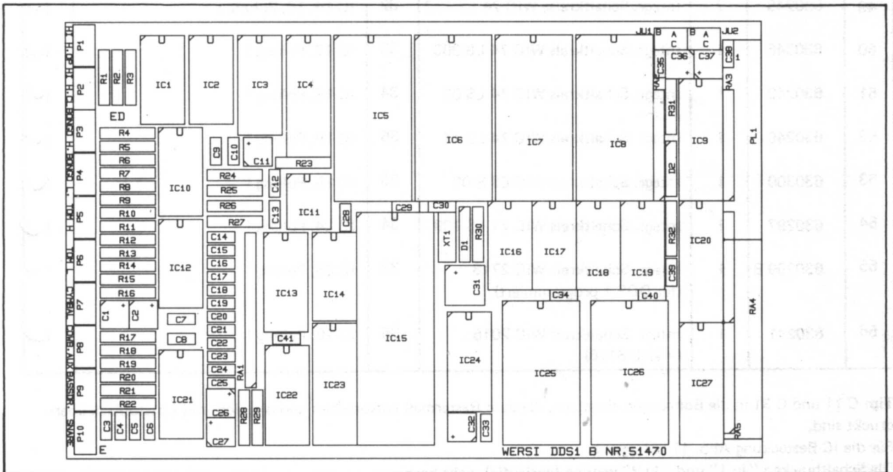
Abb. 11: Positionsdruck DDS 1
