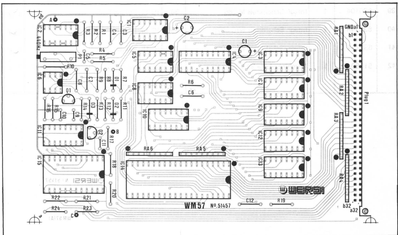
Abb. 39: Positionsdruck und Leiterbahnen WM 57
