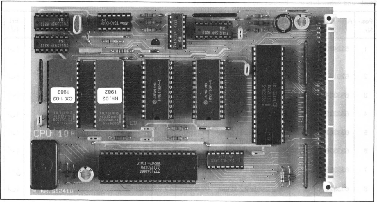
Abb. 12: Fertig bestückte Steckkarte CPU 10
