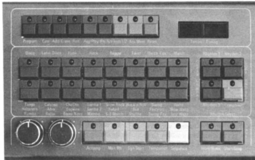
Abb. 2: Ansicht des Bedienfeldes
