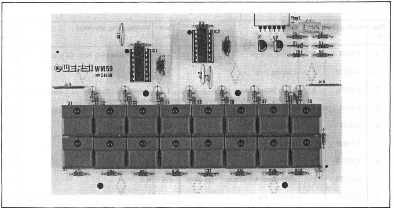
Abb. 46: Fertig bestückte Platine WM 59
