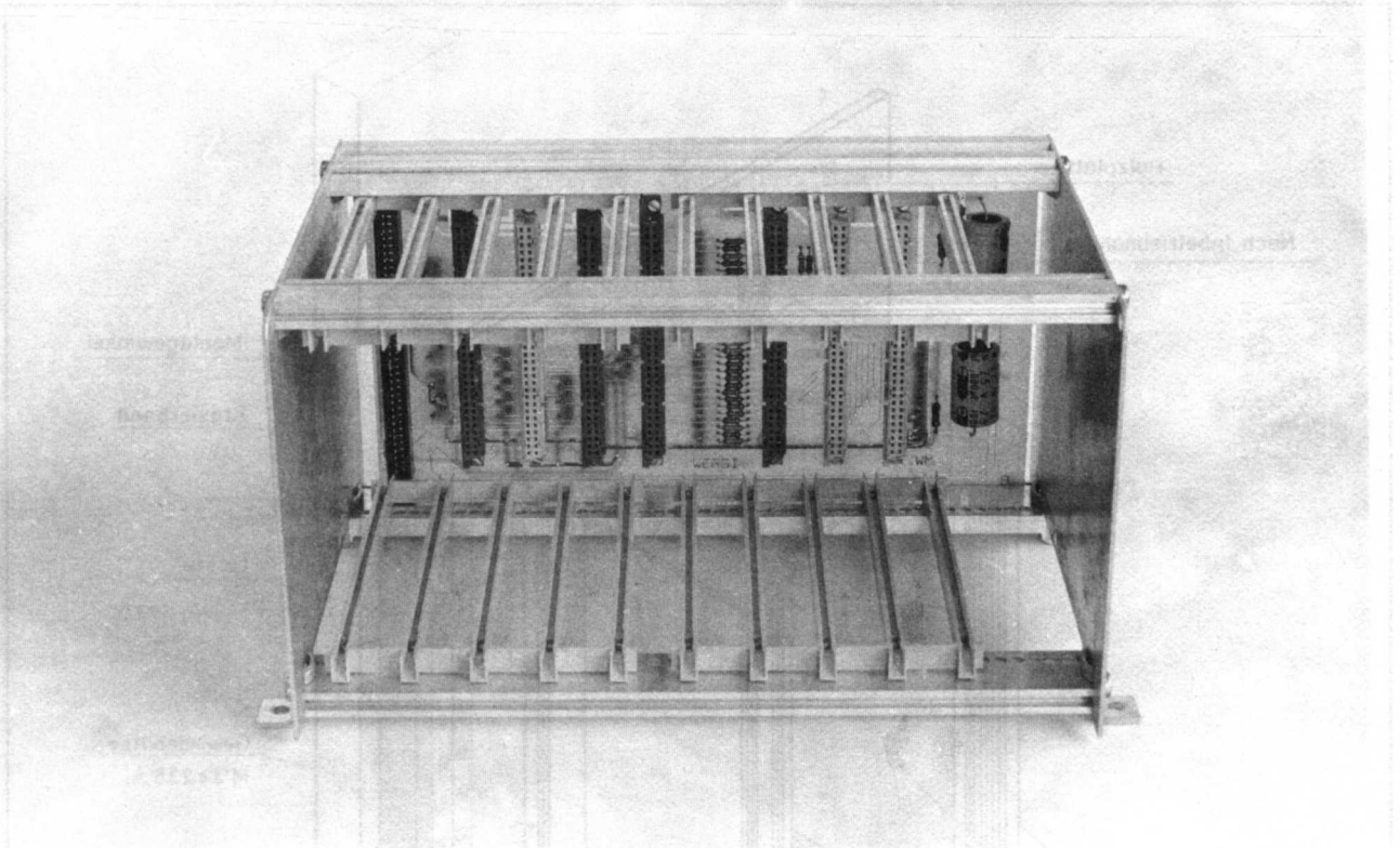
Abb. 26: Fertig montierter Baugruppenträger
