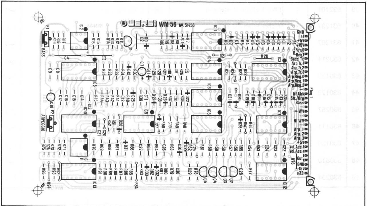
Abb. 41: Positionsdruck und Leiterbahnen WM 56
