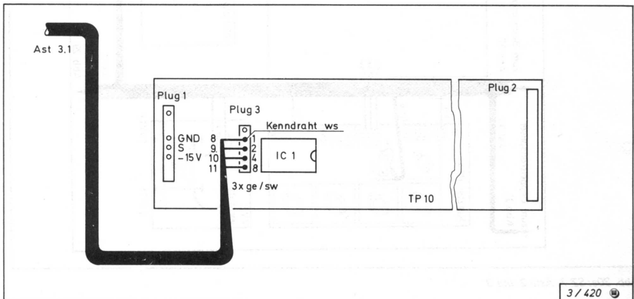
Abb. 31: SZ 6 bzw. SZ 7, Ast 3.1 am Doppeltransposer
