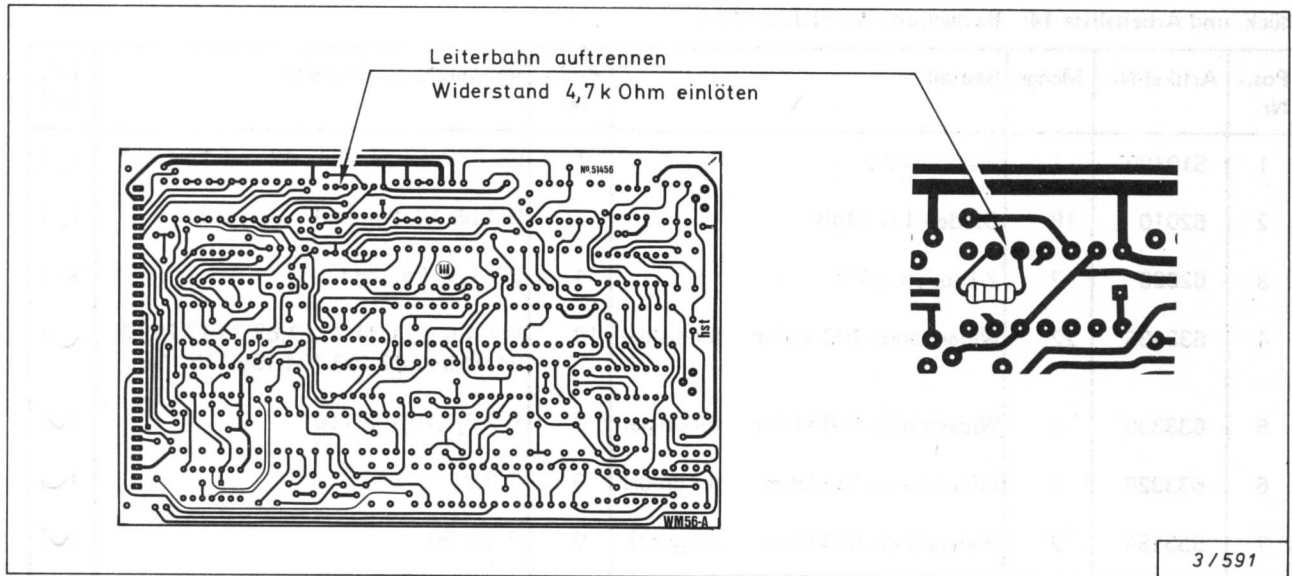
Abb. 41a: Zusatzwiderstand für WM 56
