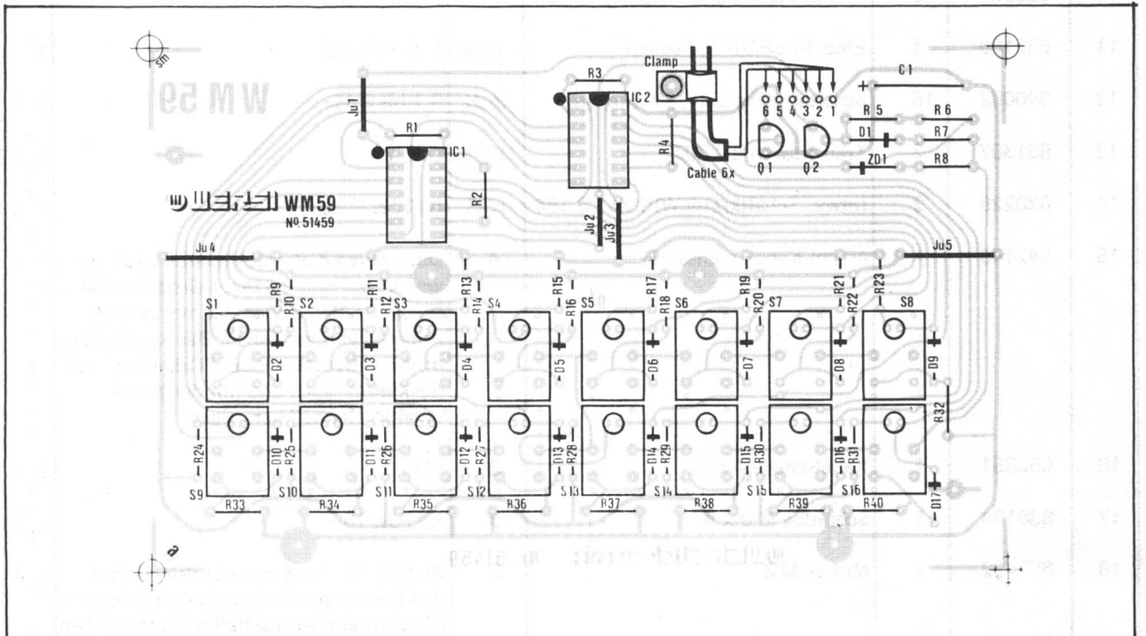
Abb. 47: Positionsdruck und Leiterbahnen WM 59
