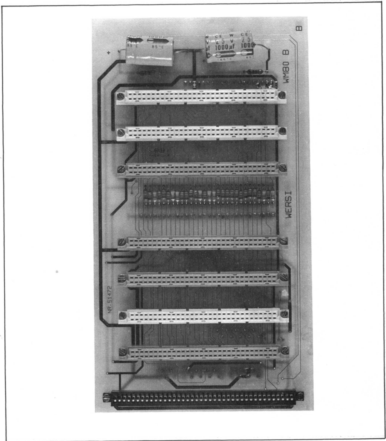
Abb. 6: Fertig bestückte Grundplatine WM 80, A-Seite
