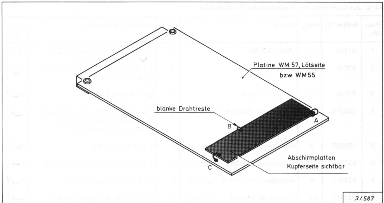
Abb. 39a: Befestigung der Abschirmplatte
