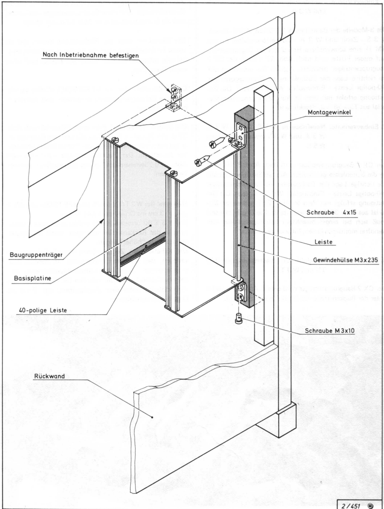
Abb. 27b: CX 2-Neueinbau in W 1 S, W 2 S, W 3 S und W 3 A
