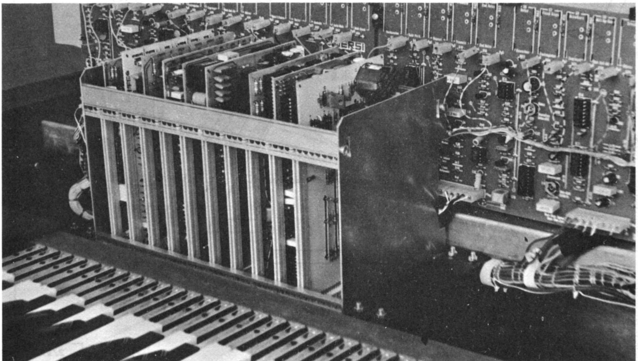
Abb. 27f: CX 2 in W 4 SKT GALAXIS
