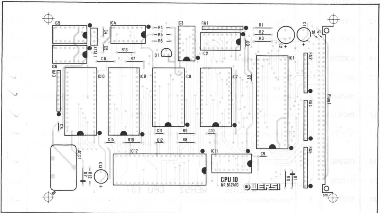
Abb. 13: Positionsdruck und Leiterbahnen CPU 10
