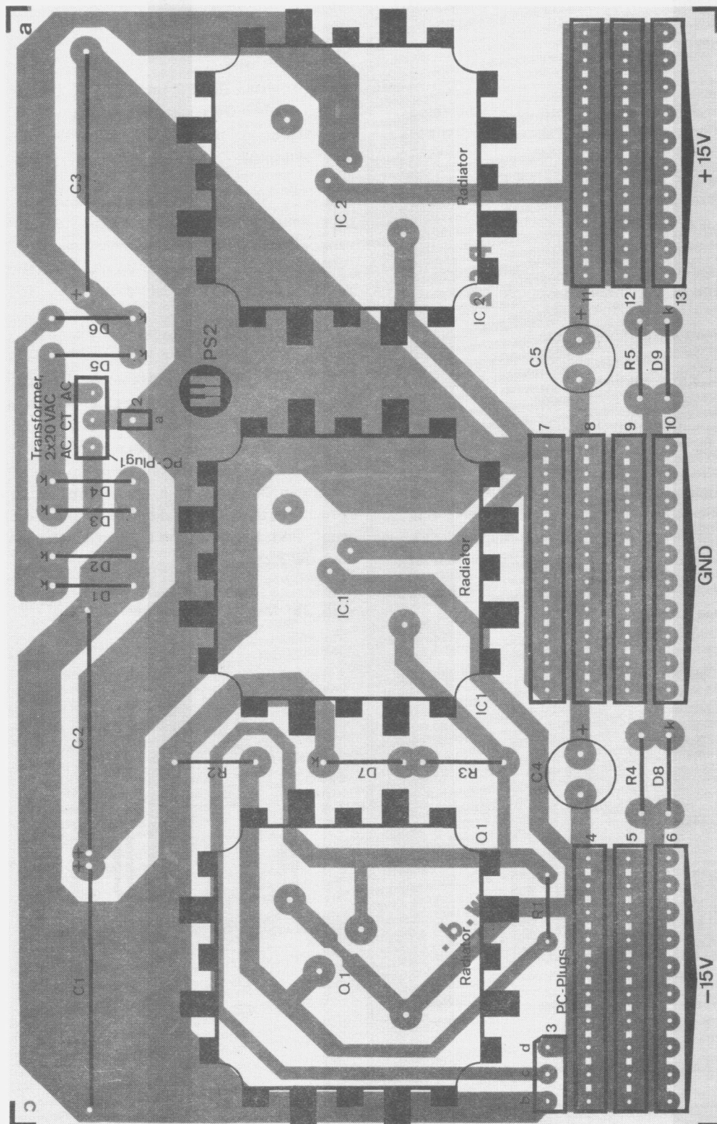
Abb. 2: Platine PS 2, Positionsdruck mit gerastert unterlegter Leiterbahn
