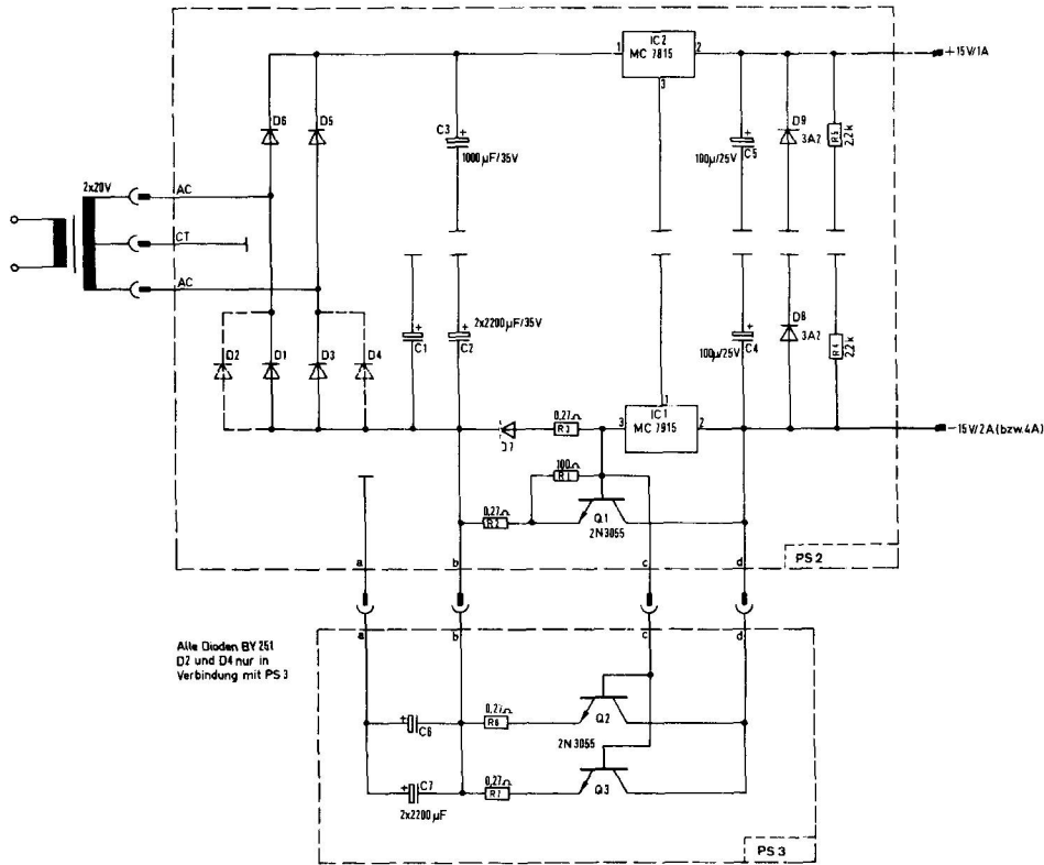
Abb. 1: Schaltung des Netzteils PS 2 und des Zusatzes PS 3
