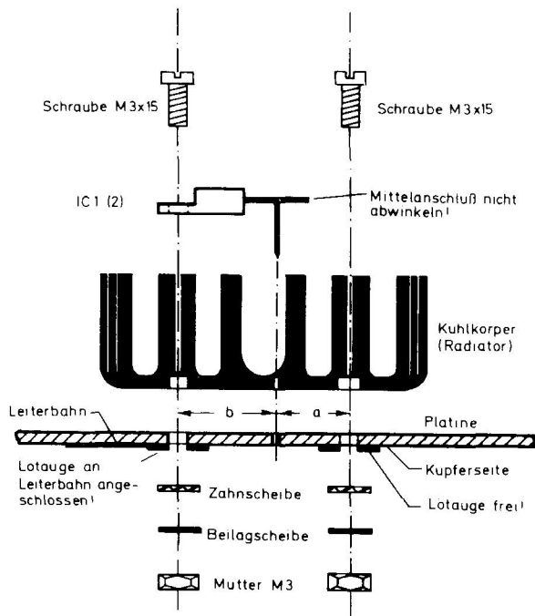
Abb. 3a: Montage der ICs
