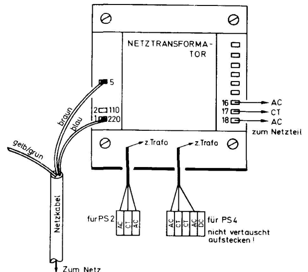
Abb. 6: Netztransformator
