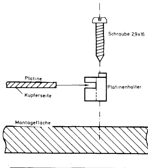
Abb. 8: Befestigung der Platine
