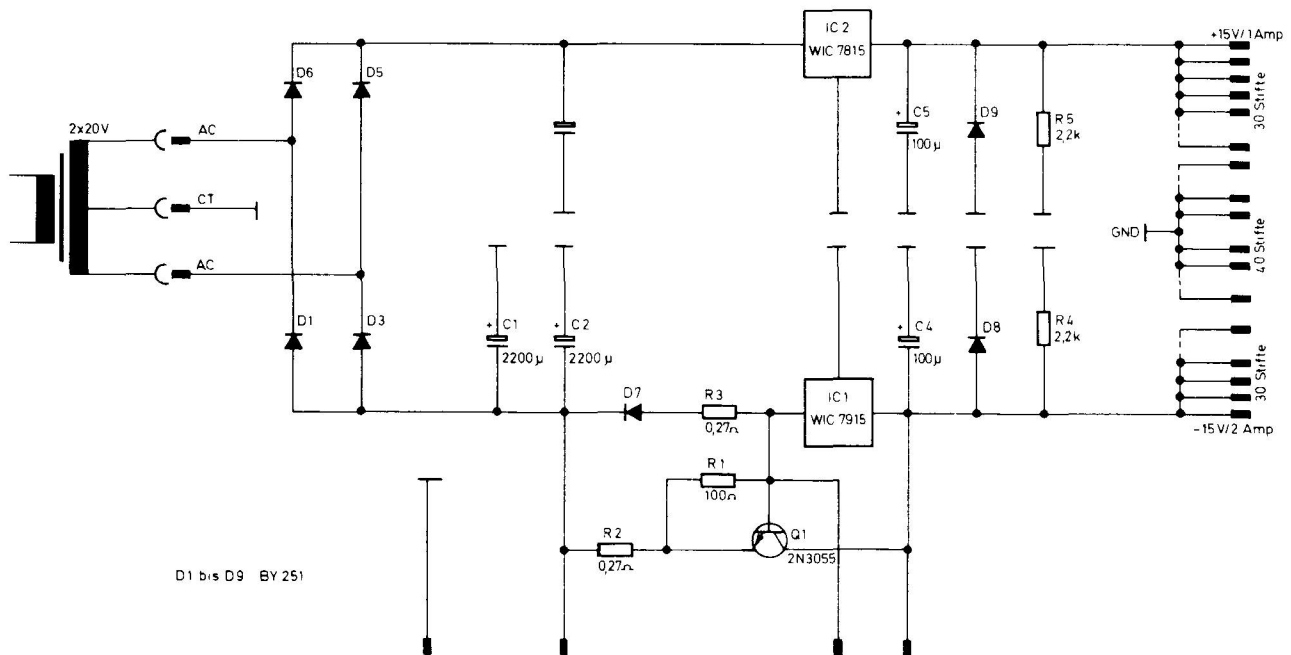
Abb. 1: Schaltung des Netzteils PS 2
