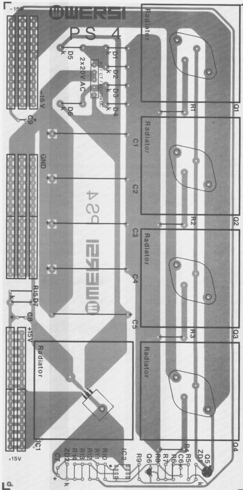
Abb. 5: Platine PS 4, Positionsdruck mit gerastert unterlegter Leiterbahn
